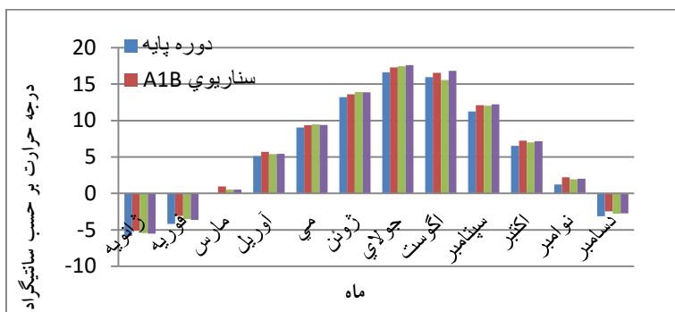
شکل ۶: میانگین دمای حداقل دوره‌ی پایه (۱۹۹۲-۲۰۰۹) و مدل IPSL4CM3 تحت تاثیر سه سناریوی A1B و A2 و B1
