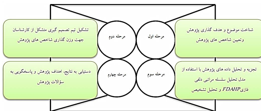
شکل ۱: مدل مفهومی فرآیند انجام پژوهش
