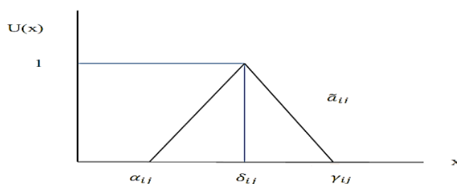
شکل ۲: تابع عضویت مثلثی در روش دلفی فازی
