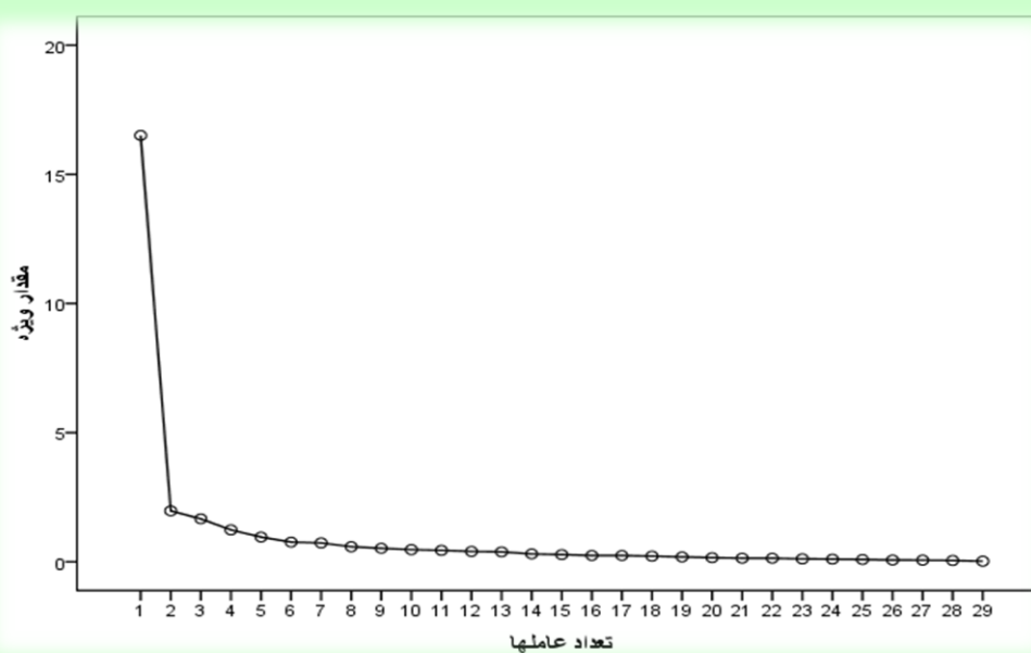
شکل شماره ۲: نمودار سنگریزه ای برای تعیین تعداد عامل ها
