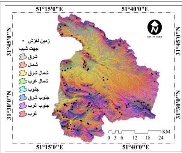
شکل ۴: جهت شیب
