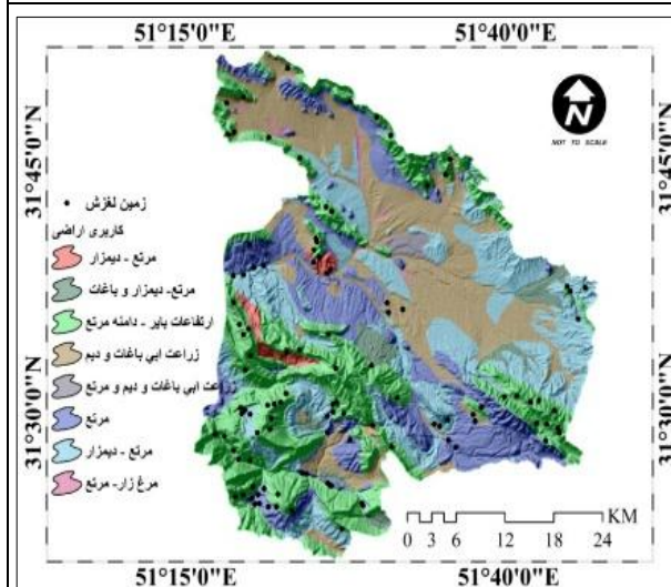
شکل ۹: کاربری اراضی
