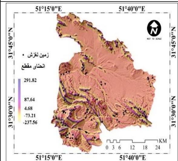
شکل ۸: انحنای مقطع
