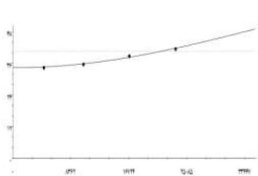
ب- مدل گوسی سیلت
