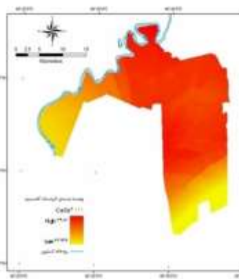
ح- پهنه‌بندی کرنات کلسیم
