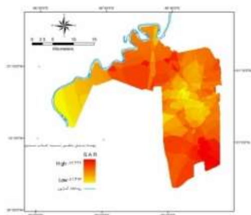
ک- پهنه‌بندی نسبت جذب سدی
