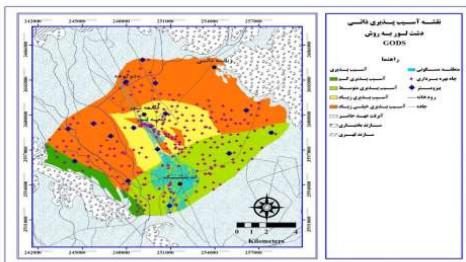
شکل ۸: نقشه آسیب‌پذیری آبخوان به آلودگی به روش GODS
