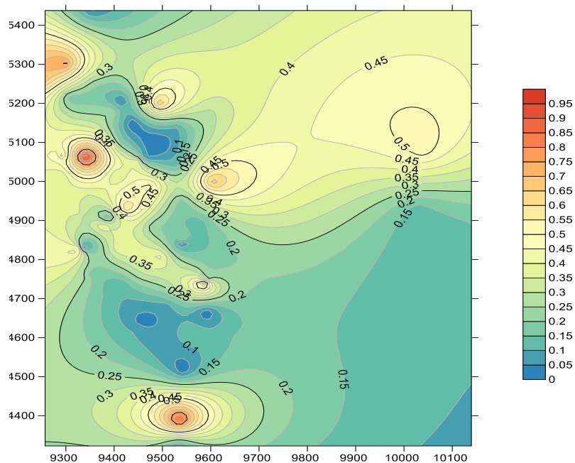
شکل ۸: میانگین درصد عیار مس به همراه گمانه‌ها و نقشه آنومالی مس در عمق بین ۳۰۰ تا ۶۰۰ متر
