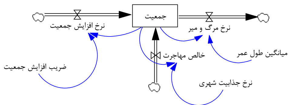
شکل ۲: زیرسیستم جمعیتی
