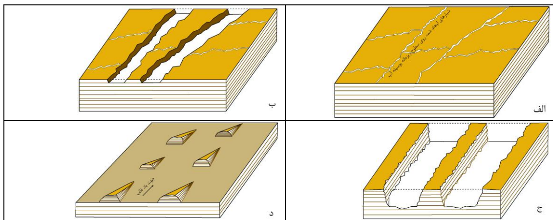
شکل ۳: الف) شروع شیارهای روی سطوح رسوبی خشک شده، ب) وسیعتر شدن شیارها بوسیله فرسایش آبی و بادی، ج) بوجود آمدن یاردانگها و د) تبدیل یاردانگها به کلوتک
