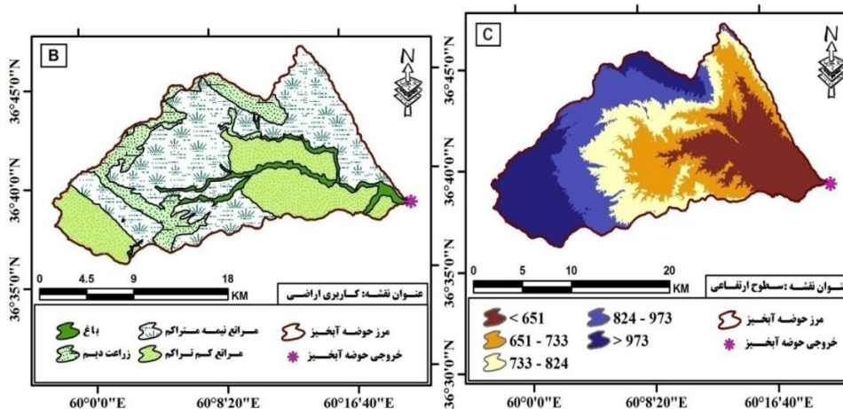
شکل ۵: عوامل ایجاد آبکندها: A: سنگ‌شناسی، B: کاربری اراضی، C: ارتفاع، D: جهت شیب، E: تندی شیب، F: شکل شیب، G: شاخص رطوبت توپوگرافی، H: تراکم زهکشی، I: فاصله از رودخانه، G: فاصله از جاده. Figure 5: Gully conditioning factors): A: lithology, B: land use, C: altitude, D: slope aspect, E: slope steepness, F: plan curvature, G: Topographic Wetness Index (TWI), H: drainage density, I: distance from rivers, G: distance from roads.
