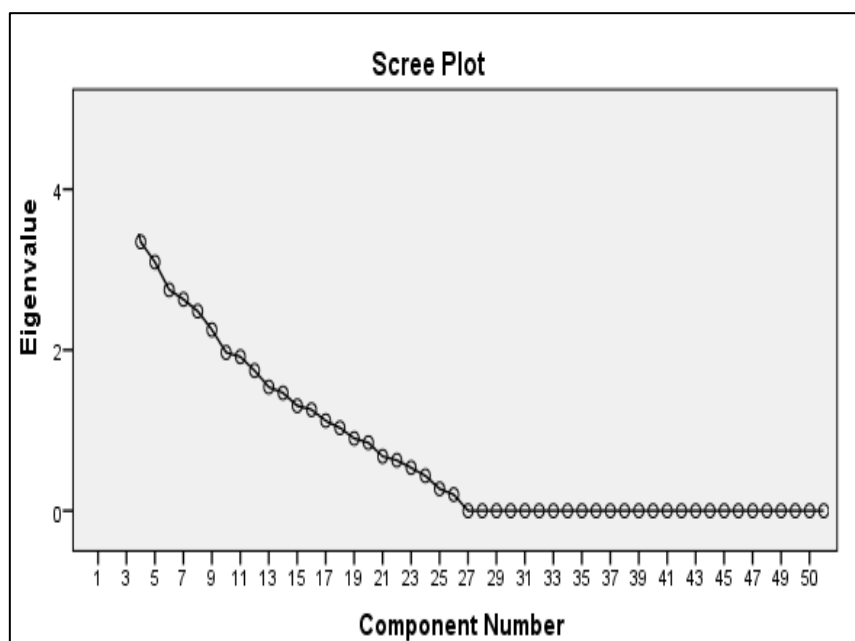
شکل ۲: نمودار اسکاتریلات
