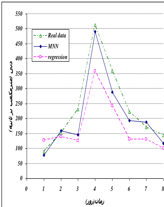
شکل شماره ۱۱- مقایسه هیدروگراف سیل خروجی و روندیابی شده با مدل‌های مختلف مربوط به سیلاب دی ماه ۱۳۸۸
