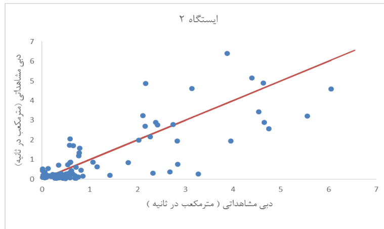
شکل ۵: دبی‌های مشاهده‌ای و شبیه‌سازی شده برای دوره صحت‌سنجی در ایستگاه دو
