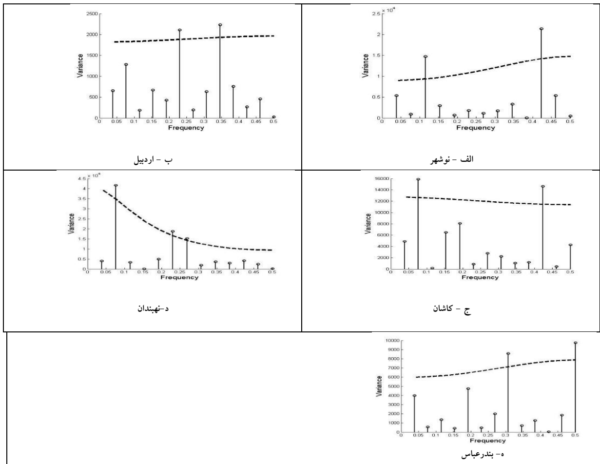
شکل ۲: دوره نگاره‌های چرخه‌های معنی‌دار (۹۵٪) ایستگاه‌های منتخب (الف ناحیه ۱ بسیار دیرپا، ب ناحیه ۲ دیرپا، ج ناحیه ۳ میان‌دوره، د ناحیه ۴ کوتاه، ه ناحیه ۵ بسیار کوتاه فصل بارش کشور در دوره مرطوب (سپتامبر - می) سال‌های ۲۰۱۵-۱۹۹۰
