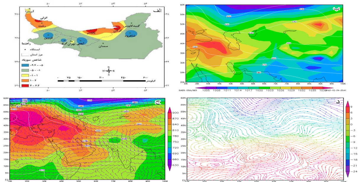
شکل ۱۲: الف- الگوی مکانی شاخص سوزباد، ب- هم‌دید تلفیقی فشار سطح دریا و ارتفاع ژئوپتانسیل تراز ۵۰۰ هکتوپاسکال، ج- هم‌دید تلفیقی ارتفاع ژئوپتانسیل ترازهای ۷۰۰ و ۹۲۵ هکتوپاسکال و بردار باد تراز ۷۰۰ هکتوپاسکال، د- وزش دمایی تراز ۷۰۰
