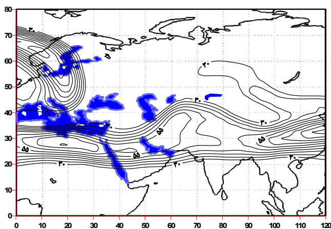
D: سرعت رودباد ۲۵۰ هکتوپاسکال به 10^{-4} \text{ g} \cdot \text{kg}^{-1} \cdot \text{s}^{-1}
