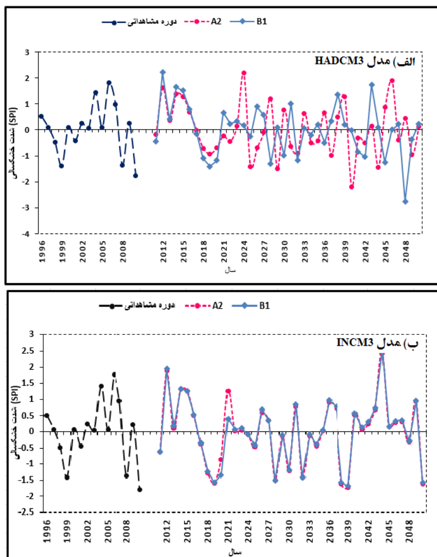
شکل ۶: خشکسالی‌های سالانه ایستگاه الیگودرز برای دوره‌ی (۲۰۵۰-۲۰۴۰) و دوره‌ی مشاهداتی (۱۹۹۶-۲۰۱۰)
