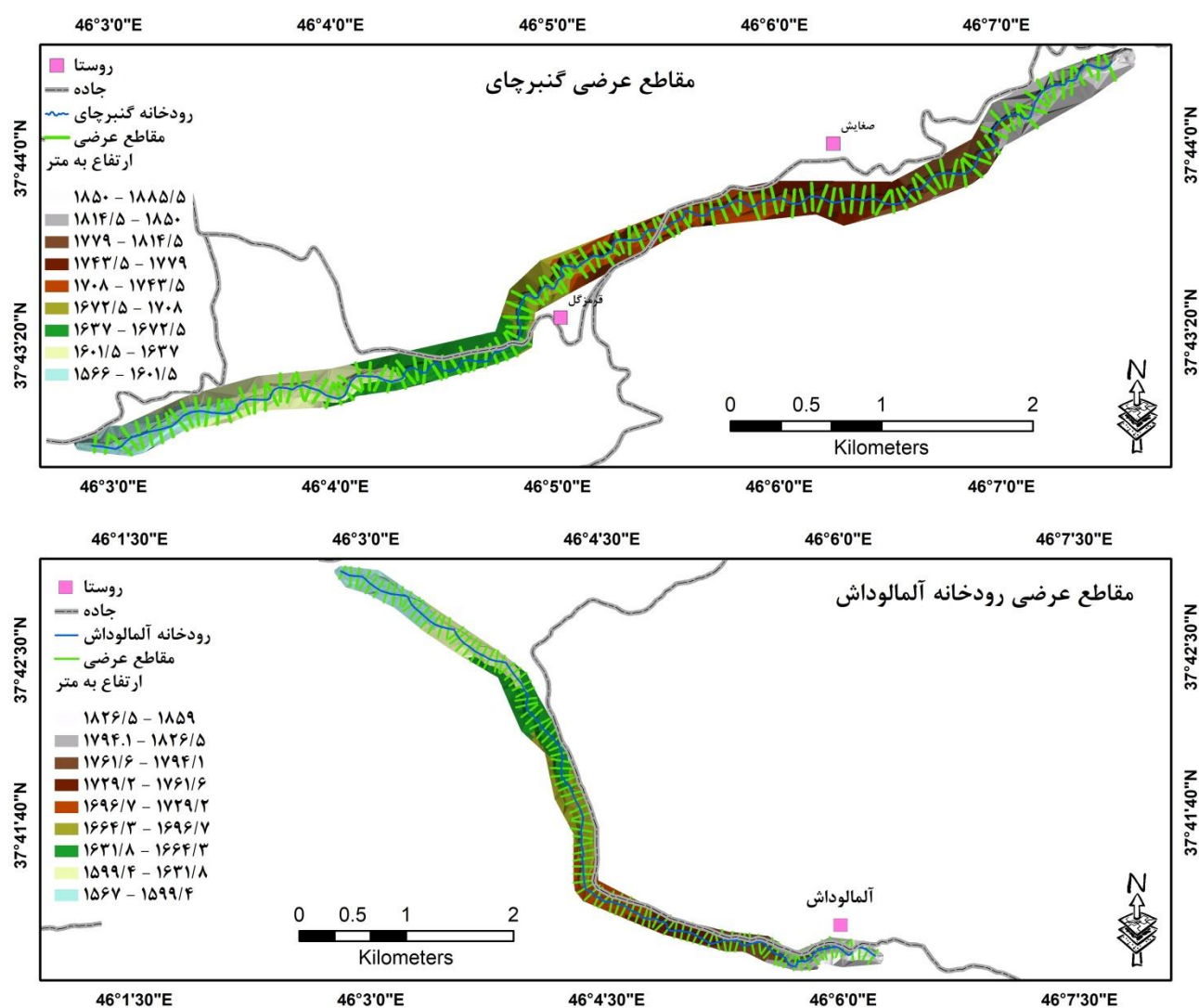
شکل ۲- مشخصات هندسی رودخانه‌های گنبرچای و آملوداش در محیط نرم‌افزاری GIS
