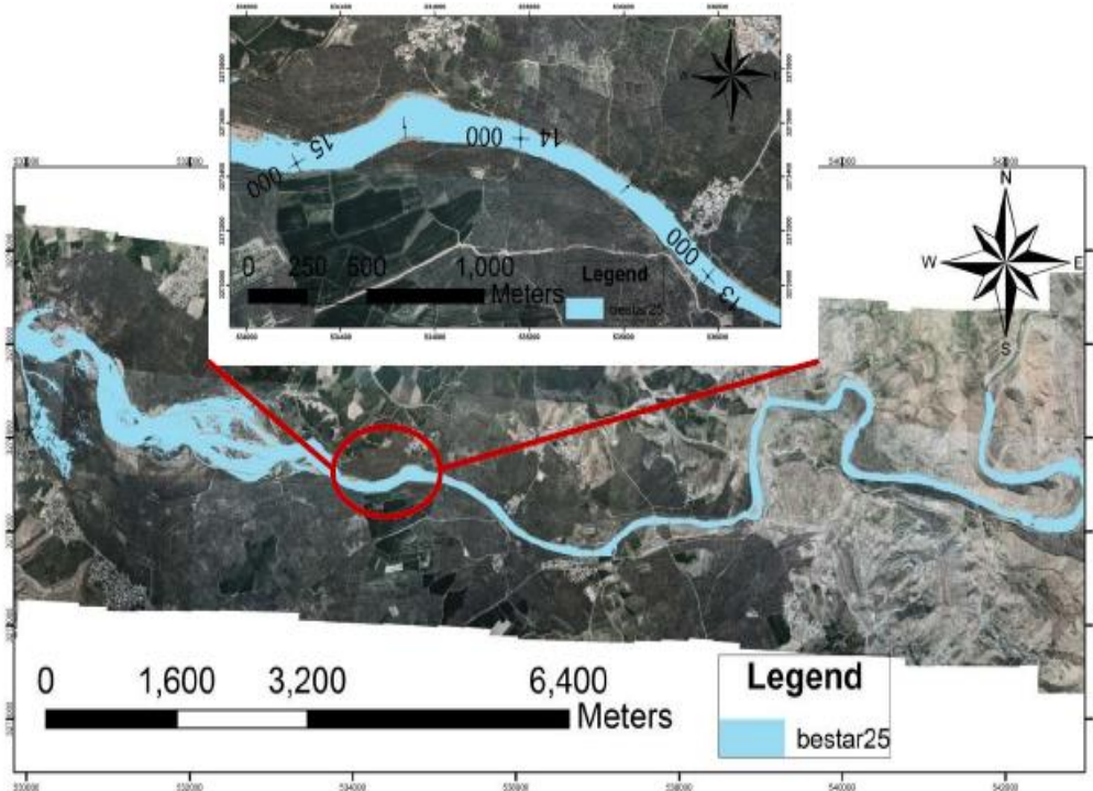
شکل ۱۶: پهنه‌ی سیلاب رودخانه‌ی شاپورخست با دوره بازگشت ۲۵ سال
