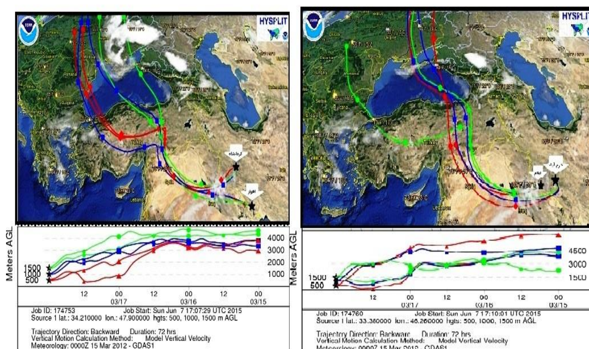
شکل ۷: خروجی مدل HYSPLIT در Google Earth و ردیابی پسگرد توفان گردوغبار توفان سوم
