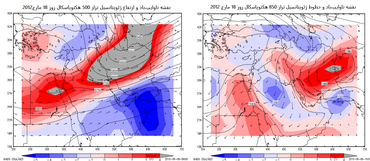
شکل ۸: نقشه‌های ژئوپتانسیلی، تاوایی و بادی در سطوح ۵۰۰ و ۸۵۰ هکتوپاسکال روز ۱۸ مارس ۲۰۱۲ (توفان سوم)
