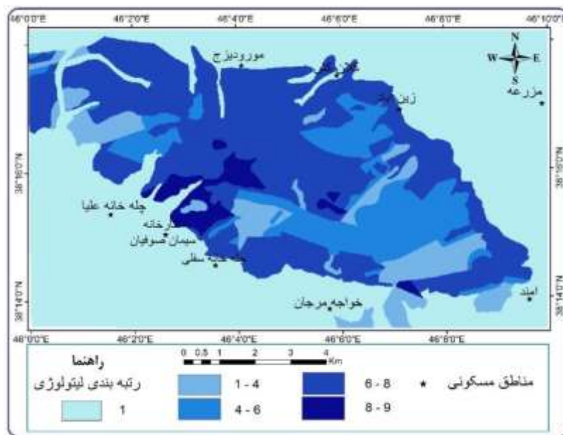
شکل ۳: نقشه رتبه‌بندی واحدهای زمین‌شناسی
