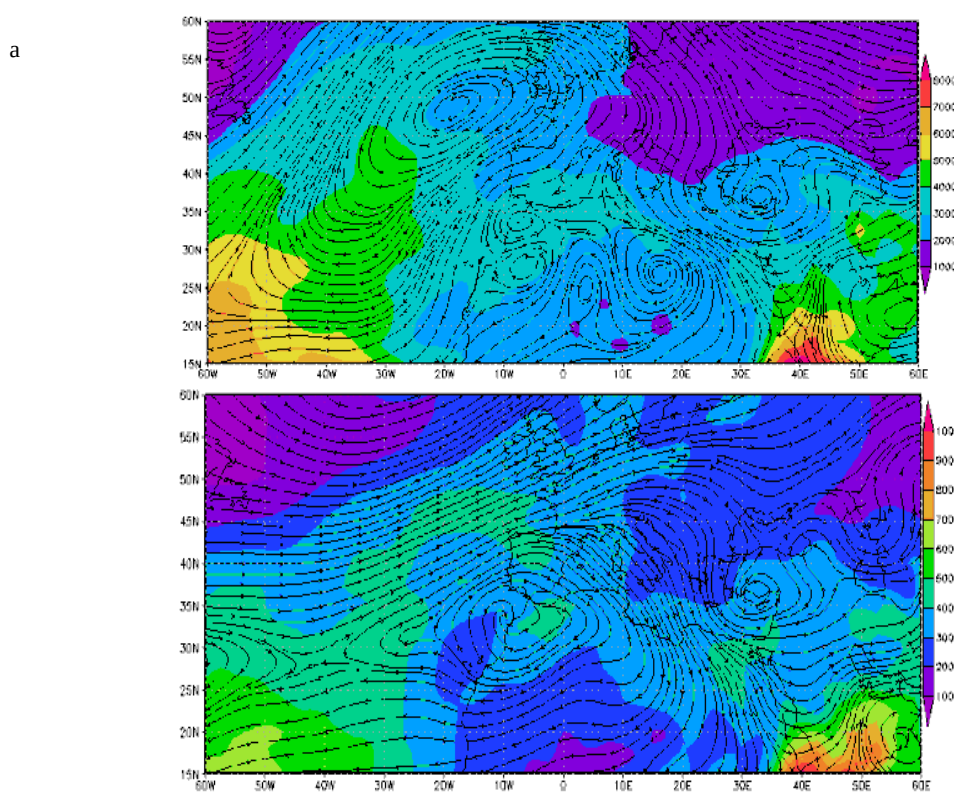
شکل ۱۵: وزش رطوبت در تراز ۸۵۰ هکتوپاسکال = فاز منفی و b = فاز مثبت
