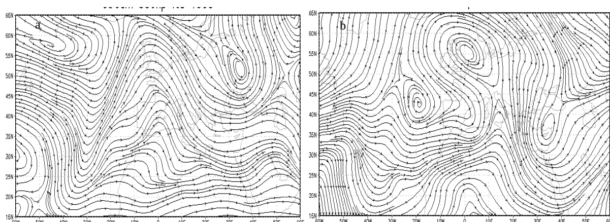
شکل ۱۴: جریان هوا در تراز ۵۰۰ هکتوپاسکال = فاز منفی و b = فاز مثبت
