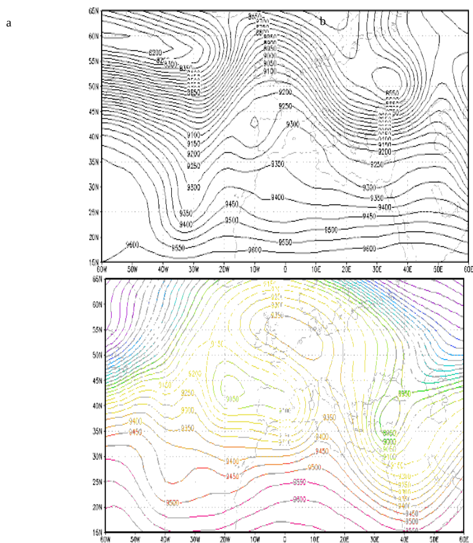
شکل ۱۲: ارتفاع ژئوپتانسیل تراز ۳۰۰ هکتوپاسکال a= فاز منفی و b= فاز مثبت
