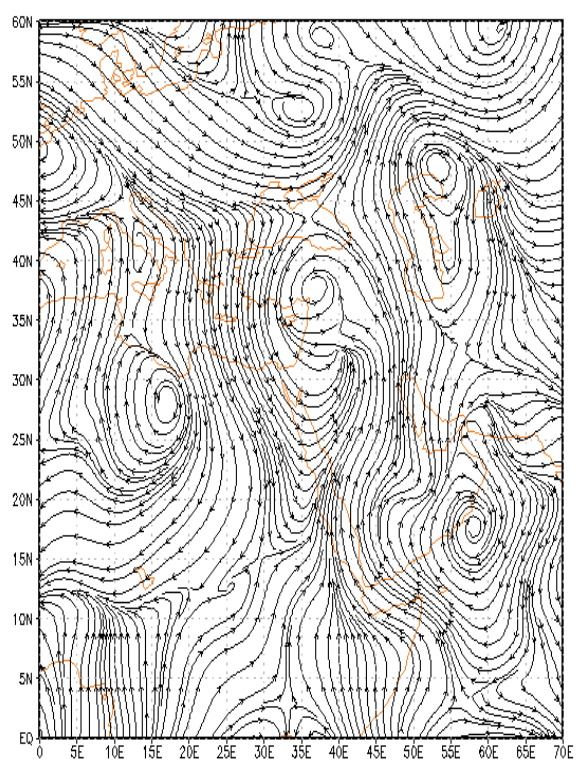
شکل ۹: میدان باد در تراز ۸۵۰ هکتوپاسکال ساعت ۱۲
