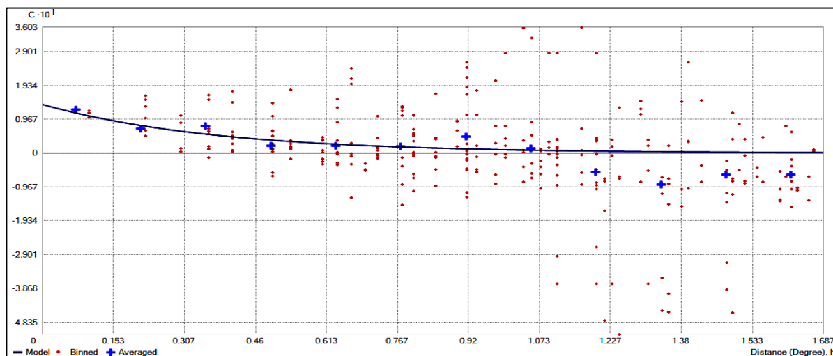
شکل ۵: منحنی نیم تغییرنمای متقابل محاسبه شده‌ی روش کوکریجینگ با مدل تنورکی برآزش داده شده به آن
