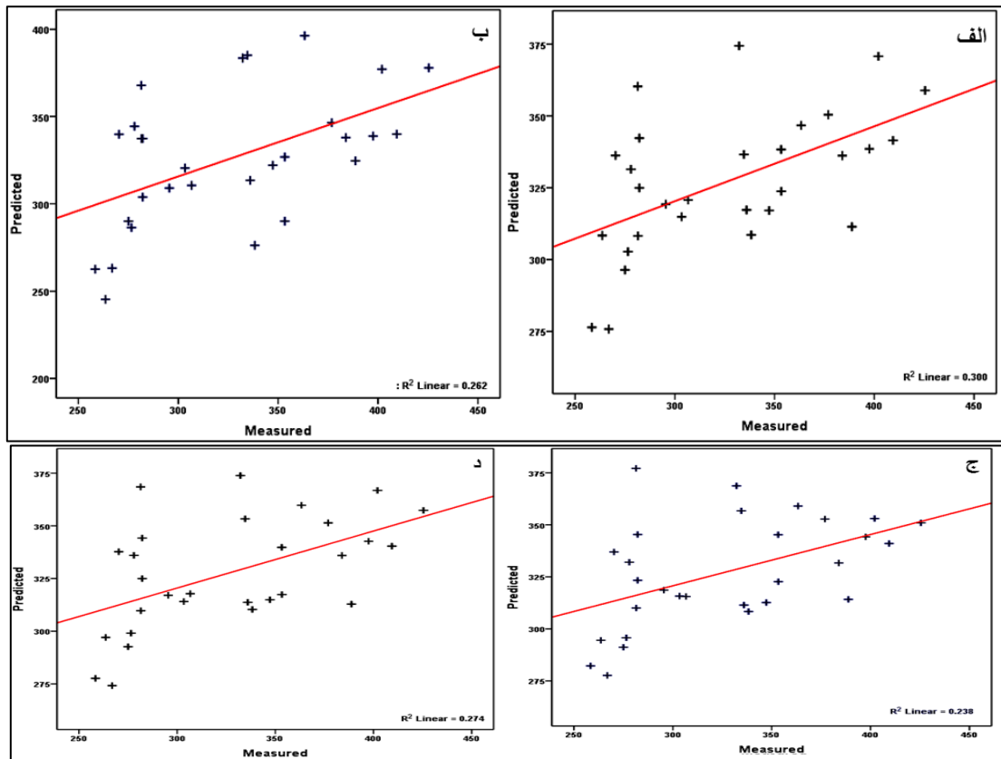
شکل ۷: نمودار پراکندگی مقادیر برآوردی و مشاهده ای چهار روش الف: کریجینگ، ب: Co کریجینگ، ج: IDW، د: Inverse Multiquadric
