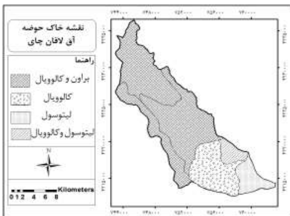
شکل ۱۱: نقشه خاک Figure 11: Soil map
