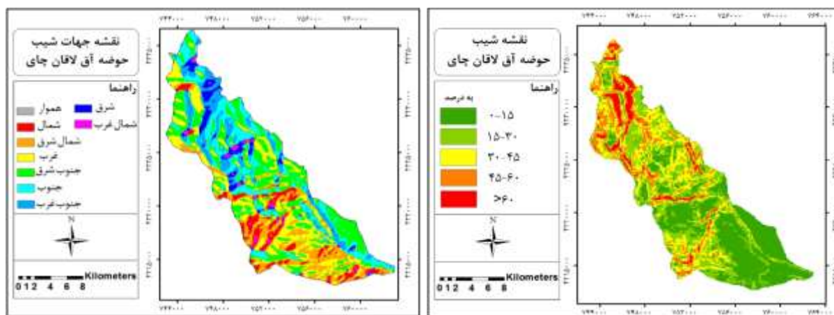
شکل ۶: نقشه شیب
