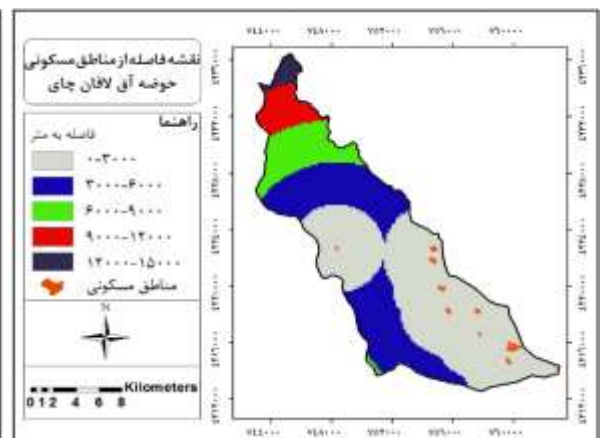
شکل ۱۰: نقشه فاصله از مناطق مسکونی Figure 10: Distance from residential area map
