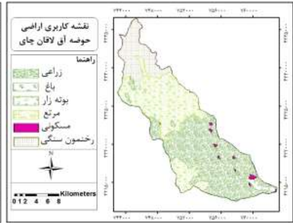
شکل ۸: نقشه کاربری اراضی Figure 8: Landuse map
