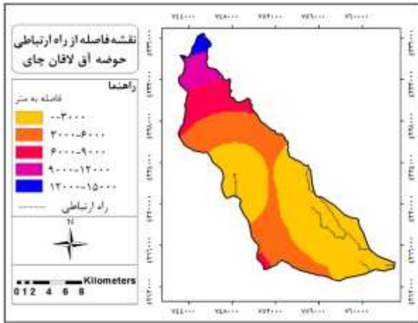
شکل ۹: نقشه فاصله از راه ارتباطی Figure 9: Distance from roads
