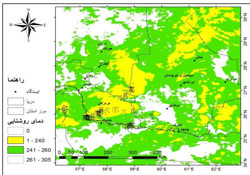
شکل ۸: دمای روشنایی باند ۴ سنجنده AVHRR در تاریخ ۰۵ ژانویه ۲۰۰۸ ساعت ۰۵:UTC06 به همراه داده‌های حاصل از سنجنده LIS در ساعت ۰۴:۳۴ UTC
