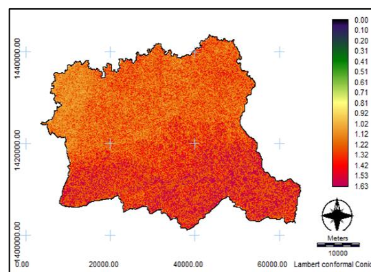
شکل ۶: نقشه عامل طول شیب (L)
