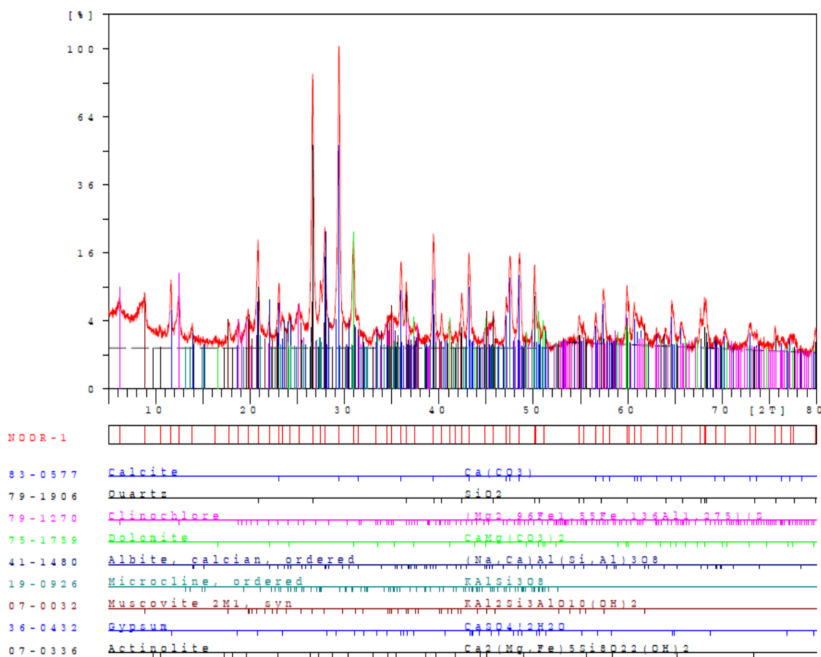
شکل ۳: نتایج تشخیص XRD از نمونه مرکب جمع آوری شده از ریزگردهای ورودی به مناطق مورد مطالعه
