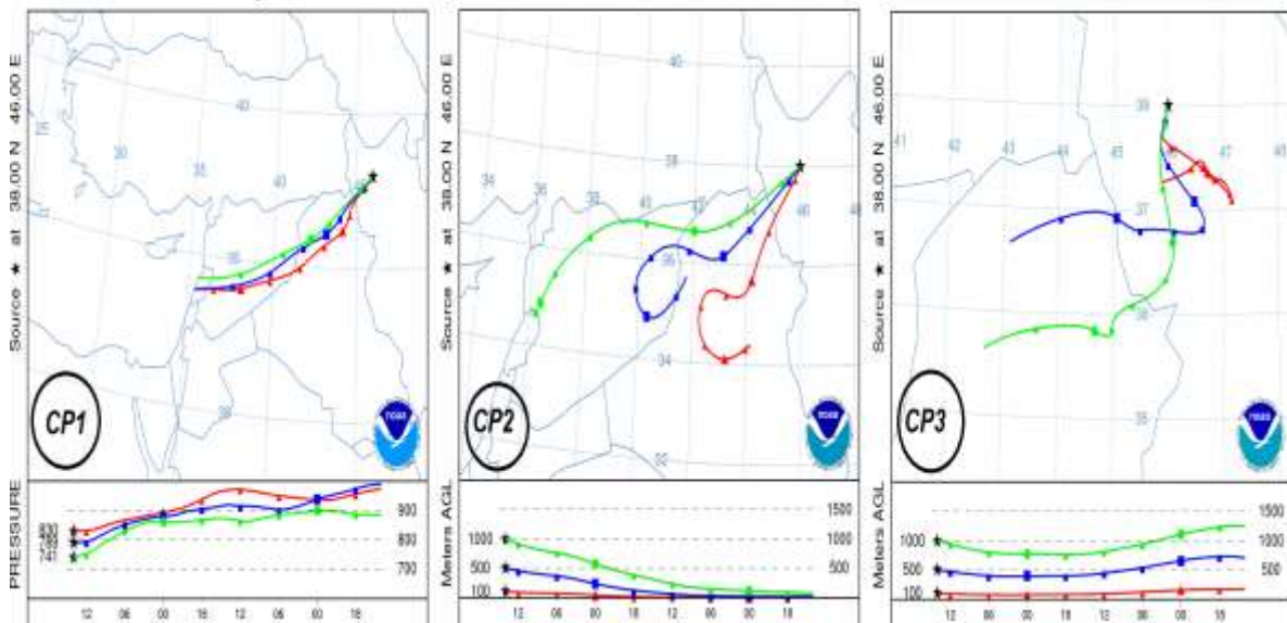
شکل ۶: ردیابی ذرات معلق با استفاده از مدل HYSPLIT در هر الگو گردشی
