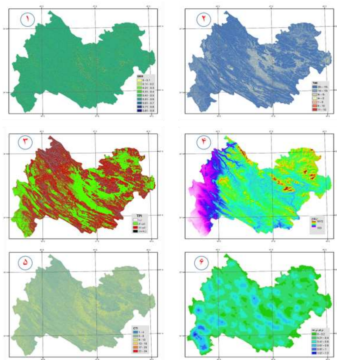
شکل ۳: لایه ژئوهیدرولوژی مستخرج از ۳۰ متر استان کرمانشاه: ۱- SRR، ۲- TWI، ۳- TPI، ۴- ارتفاع، ۵- CTI و ۶- تراکم آبراهه Figure 3: Geohydrology layer extracted of 30 m DEM of Kermanshah Province: 1- SRR, 2- TWI, 3- TPI, 4- Height, 5- CTI, 6- Condensation Channel
