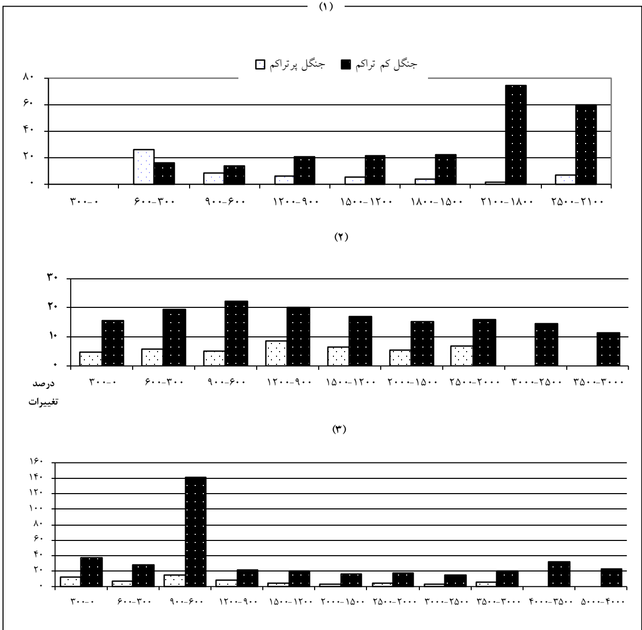
شکل ۴: درصد تغییرات (محور عمودی) هر یک از کلاسها نسبت به سطح اولیه در سال (۱۳۶۹) در هر یک از طبقات متغیرهای ارتفاع به متر (۱)، فاصله از جاده به متر (۲)، فاصله از مسکونی به متر (۳)، طبقات جهت (۴)، طبقات شیب به درصد (۵)
