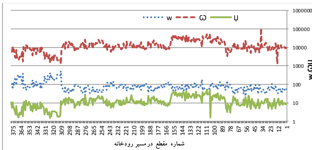
شکل ۱۲: مقایسه پهنای، قدرت برش و جریان رسوبات در مسیر رودخانه ارس Figure 12: Comparison of the width, cutting power and flow of sediments along the river Aras
