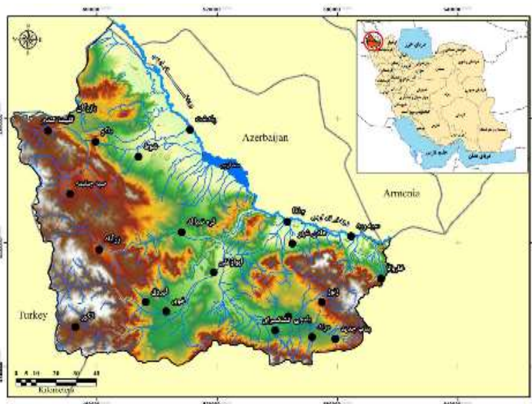
شکل ۱: موقعیت محدوده مورد مطالعه در قسمت شمال غرب ایران
