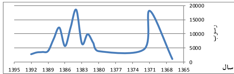
شکل ۱۱: تغییرات در میزان رسوب سالانه ارس از سال ۱۳۶۵ تا ۱۳۹۲ Figure 11: Changes in the annual precipitation rate of Aras from 1365 to 1392
