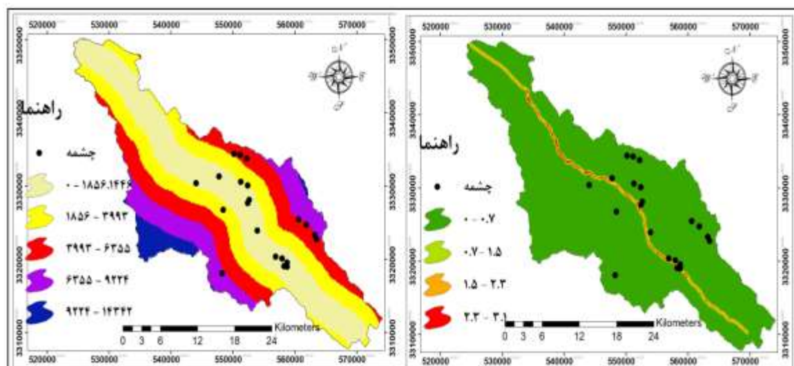
شکل ۵: الف) لایه تراکم آبراهه حوضه آبریز نورآبادممنسی، ب) لایه فاصله از آبراهه حوضه نورآباد ممسنی
