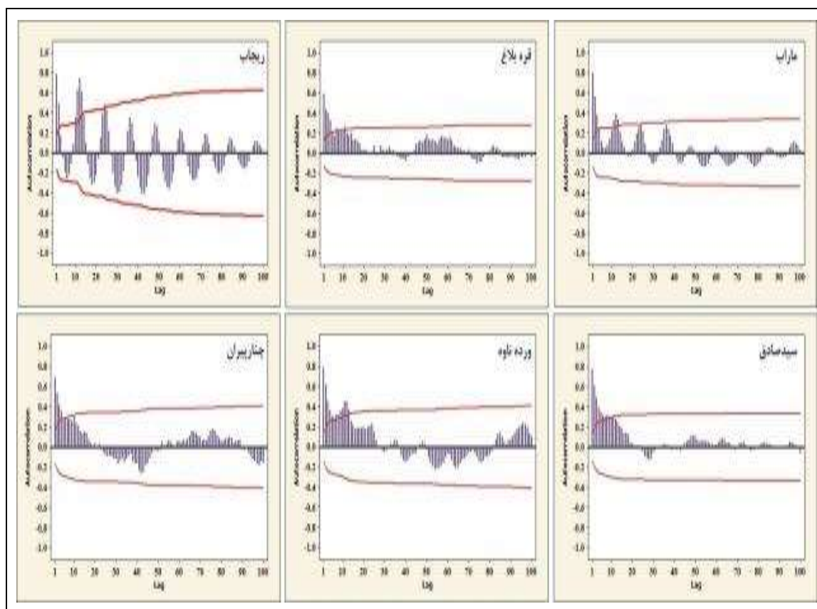
شکل ۵: کورولوگرام چشمه‌های ریجاب، قره‌بلاغ، ماراب، چنارپیران، ورده ناوه و سید صادق
