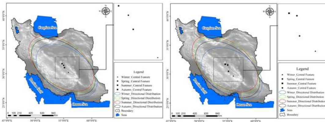
شکل ۷: گرانی گاه و توزیع مکانی دمای مشاهداتی با استفاده از آماره توزیع جهت‌دار در ایران Figure 7: Gravity and spatial distribution of observed temperature using directional distribution statistics in Iran
