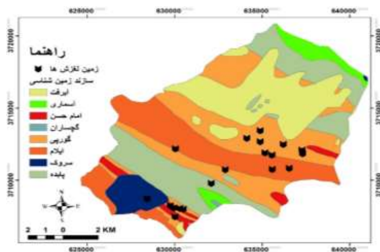
شکل ۷: همپوشانی لایه زمین لغزش و لایه زمین شناسی حوزه چاویز
