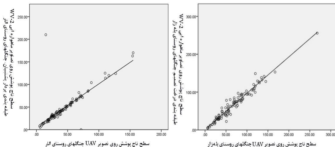
شکل ۷ الف: ارزیابی صحت سطح تاج پوشش در طبقه‌بندی بردار پشتیبان تصاویر ماهواره‌ای WV-2 و تصاویر UAV جنگل‌های روستای انار و به‌زار و انار به ترتیب از راست. به مترمربع Fig 7a: Evaluation of the accuracy of the canopy in SVM classification in satellite imagery wv-2 and UAV image in the forests of the village of Balehazar and AbeAnar. Respectively of right. To m 2
