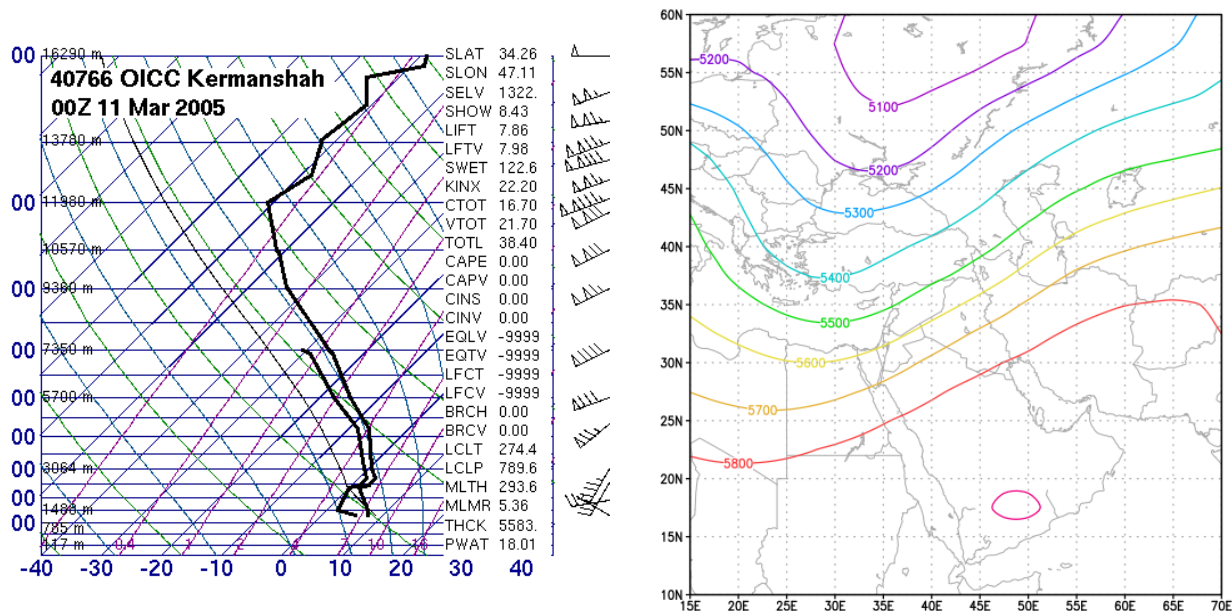
شکل ۶: نمودار Skew-T و نقشه هوا در تراز ۵۰۰ هکتوپاسکال، روز ۱۱ مارس ۲۰۰۵ (۲۱ اسفند ۱۳۸۳)
