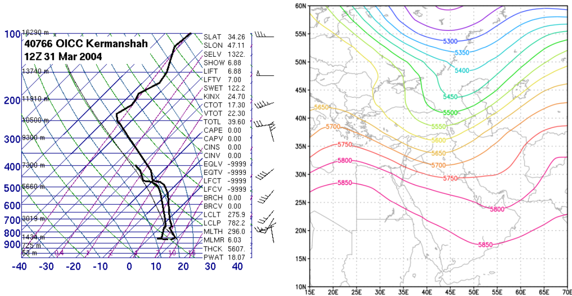
شکل ۵: نمودار Skew-T و نقشه هوا در تراز ۵۰۰ هکتوپاسکال، روز ۳۱ مارس ۲۰۰۴ (۱۲ فروردین ۱۳۸۳)
