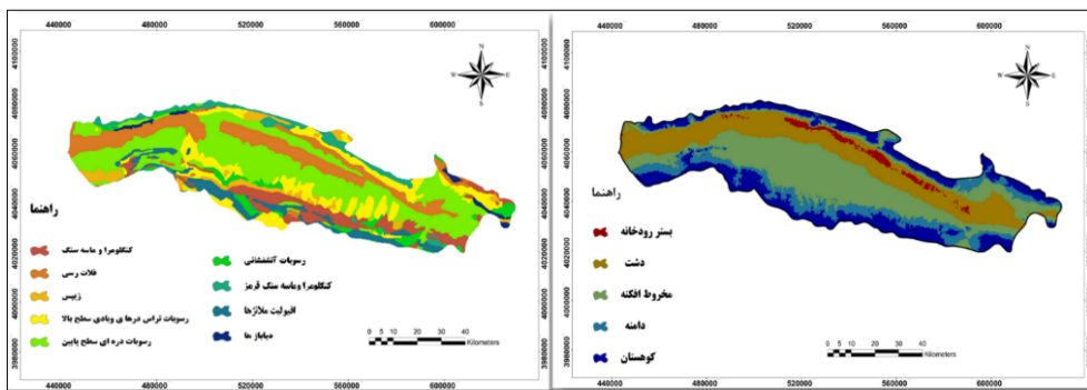
شکل ۶: الف) ژئومورفولوژی محدوده جوین؛ ب) لیتولوژی حوضه آبریز جوین Figure 6: a) Geomorphology of the Joven area, b) Lithology of the Joven catchment
