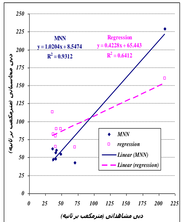
شکل شماره ۱۰- مقایسه مقادیر دبی مشاهداتی و محاسباتی حاصل از روندیابی هیدروگراف سیل با مدل های مختلف به ازای سیلاب فروردین ماه
