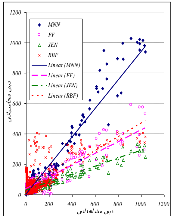
شکل شماره ۴- مقایسه دبی مشاهداتی و محاسباتی در ایستگاه پل فلور توسط مدل های EANN در مرحله آموزش
