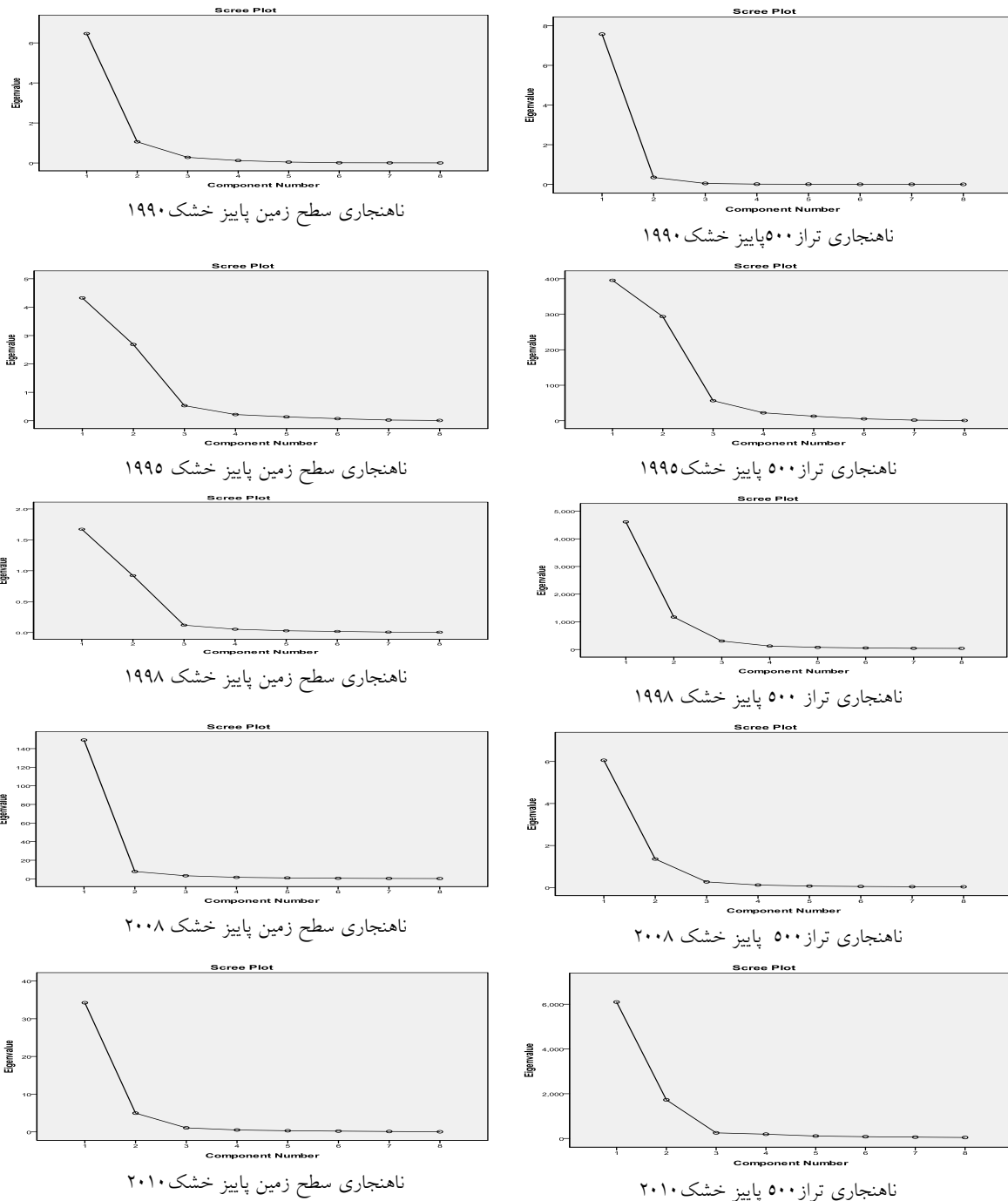
شکل ۲: نمودار ناهنجاری سطح زمین و تراز ۵۰۰ خروجی spss
