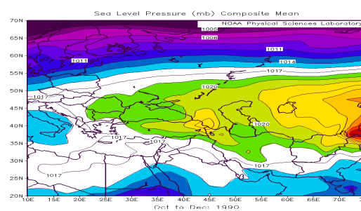
شکل ۳: نقشه فشار سطح دریا فصل خشک پاییز ۱۹۹۰
