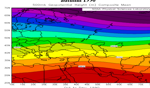
شکل ۵: نقشه تراز ۵۰۰ هکتوپاسکالی فصل خشک پاییز ۱۹۹۰
