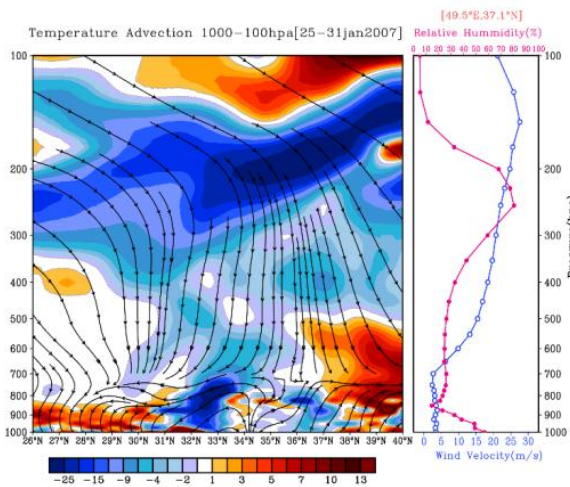
شکل ۱۲: نمودار مقطع قائم فرارفت دما برای طول ۴۹.۵ درجه شرقی و عرض ۲۶ تا ۴۰ درجه شمالی (سمت چپ)، نمودار مقطع قائم تغییرات رطوبت و سرعت باد برای نقطه ۴۹.۵ درجه شرقی و ۳۷.۱ درجه شمالی (سمت راست)-متوسط گیری شده برای کل دوره
