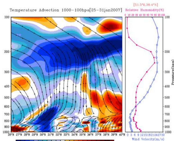
شکل ۱۳: نمودار مقطع قائم فرارفت دما برای طول ۵۱.۵ درجه شرقی و عرض ۲۶ تا ۴۰ درجه شمالی (سمت چپ)، نمودار مقطع قائم تغییرات رطوبت و سرعت باد برای نقطه ۵۱.۵ درجه شرقی و ۳۶.۴ درجه شمالی (سمت راست)-متوسط گیری شده برای کل دوره
