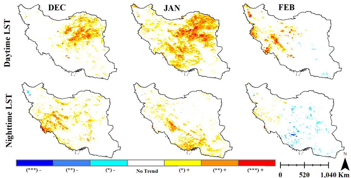
شکل ۸: روند تغییرات دمای سطح زمین در روز و شب در ماه‌های دسامبر، ژانویه و فوریه در دوره آماری ۲۰۰۳-۲۰۲۰
