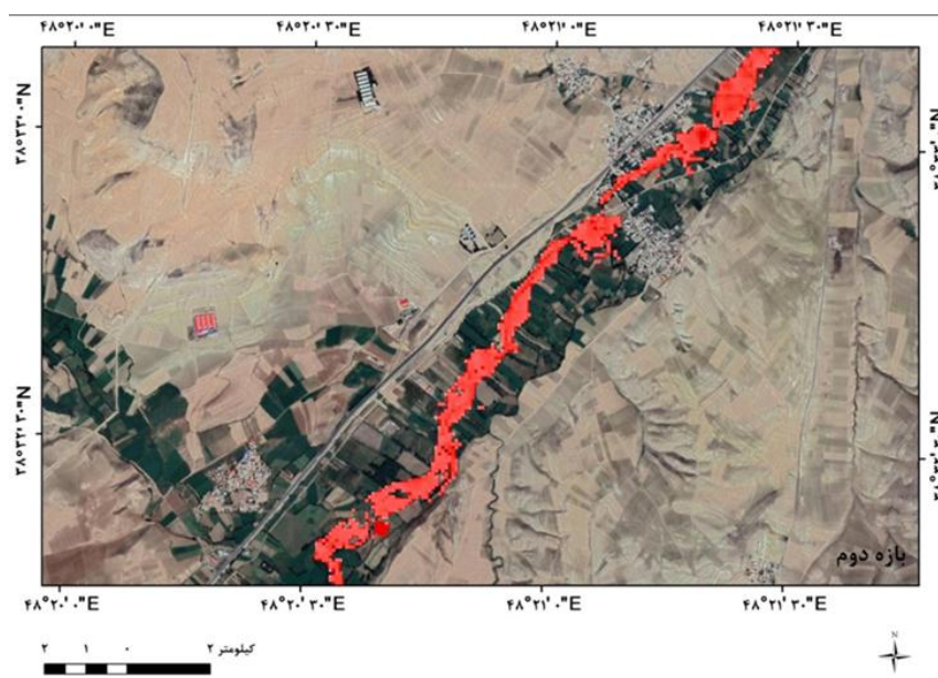
شکل ۵: پهنه‌های سیلابی رودخانه بالیخلی‌چای در بازه دوم با دوره بازگشت‌های مختلف
