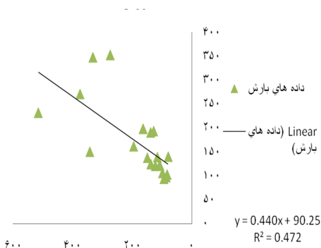
شکل شماره 8- نمودار مقایسه بارش واقعی و بارش به دست آمده به کمک GIS روش IDW
