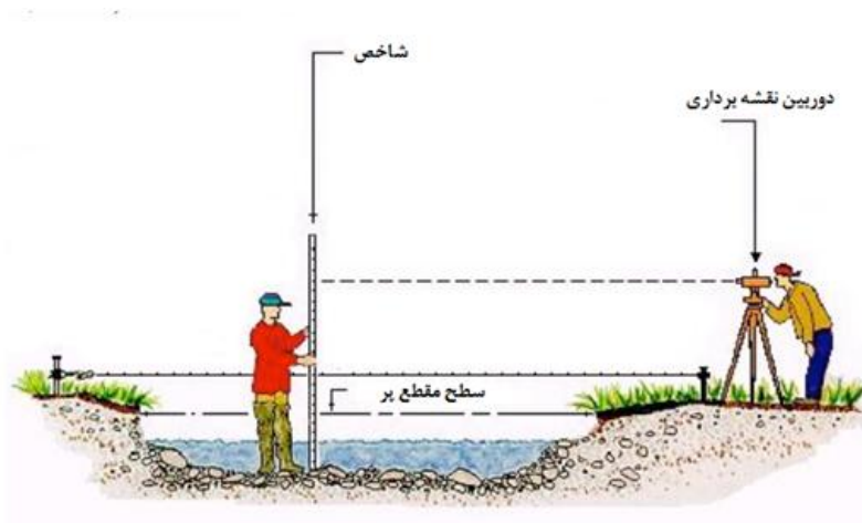
شکل ۲: سطح مقطع پر در یک مقطع عرضی اصلاح شده از راسگن ۱۹۹۶ (آربلیز و همکاران ۳ ، ۲۰۰۷: ۱۹۱)
