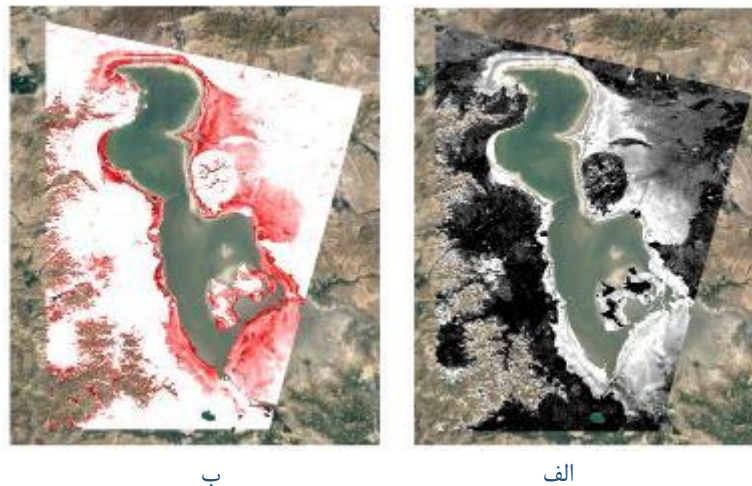
شکل ۲: الف) خروجی شاخص EC (تصویر مربوط به ۴ فروردین ۱۴۰۰)، ب) شاخص EC با یک حد آستانه جهت نمایش بهتر Figure 2: a) Output of EC index (image related to April 4, 1400), b) EC index with a threshold for better display
